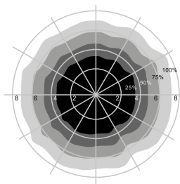
Patroon wandmontage (Eenheid: m) Voorgestelde montagehoogte: 2,5 - 6m
