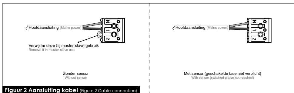
Figuur 2 Aansluiting kabel (Figure 2 Cable connection)
